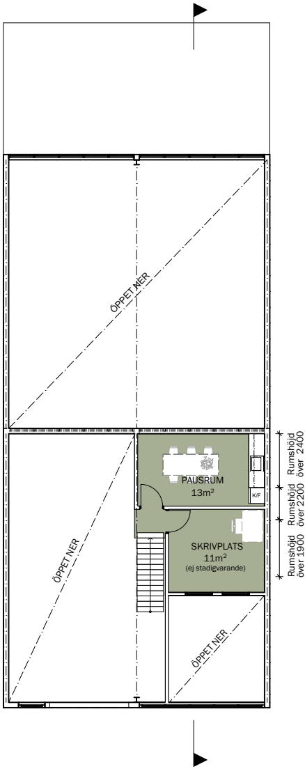
Entresolplan
