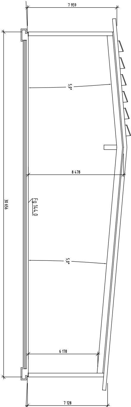
SEKTION B-B SKALA A1 1:100, A3 1:200
